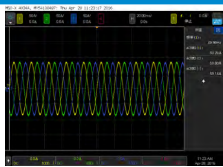
图1. 48脉波整流时的输入电流
