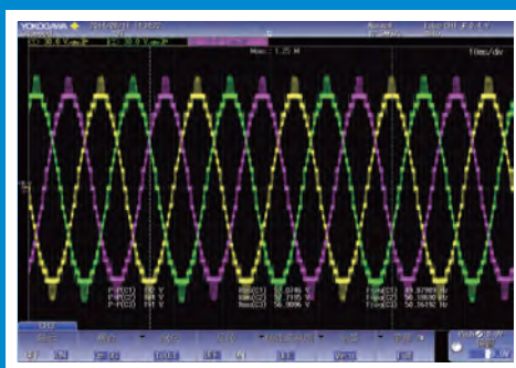
图2. 33电平输出线电压
