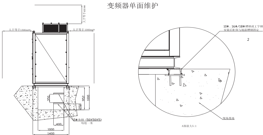
电缆沟槽及地上沟槽断面图
