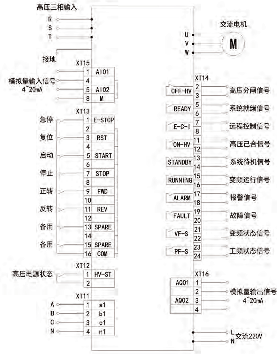
对外接线图
