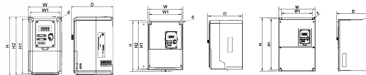
(图A)380V:1~8HP (IP20)
