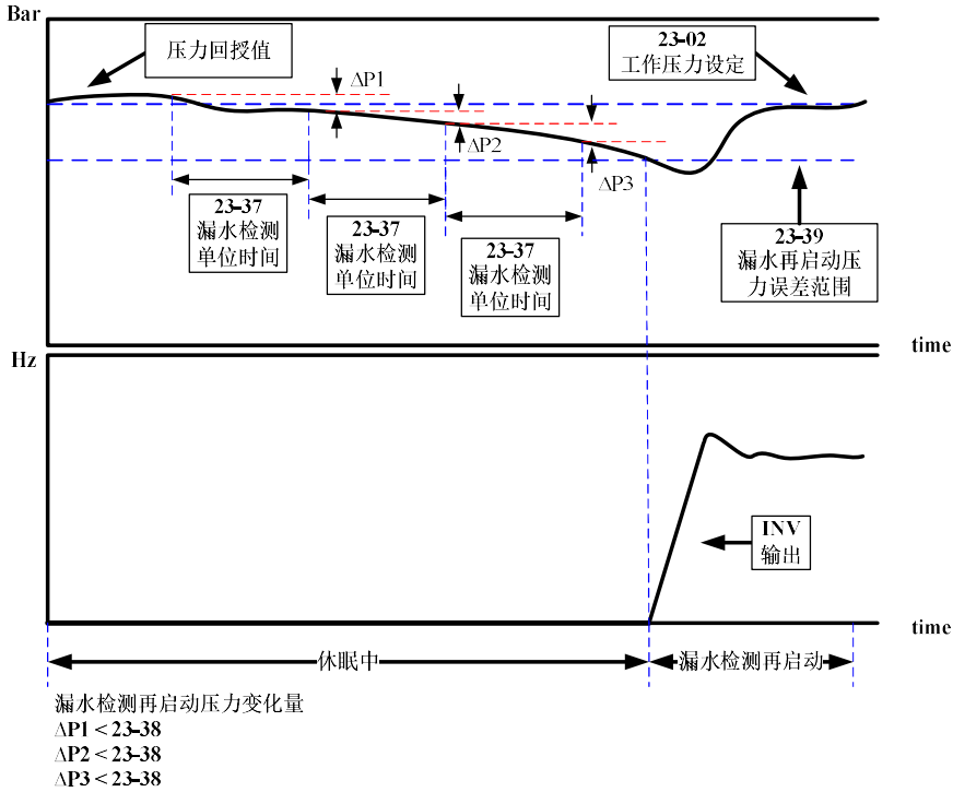
漏水检测Case2: 压力变化量小于23-38
