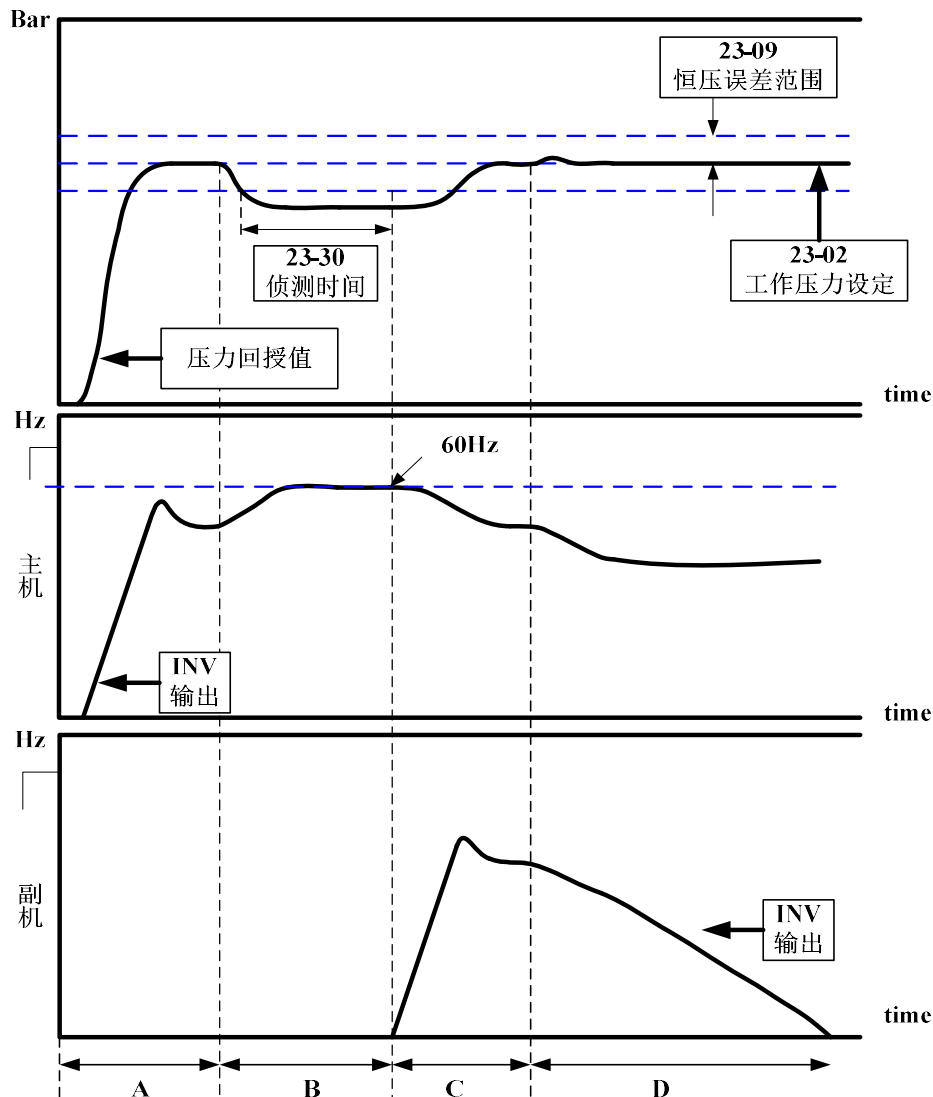
图 4.3.109 双泵浦启动功能流程
