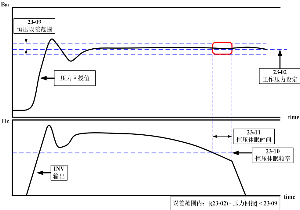
图 4.3.103 恒压停机示意图
