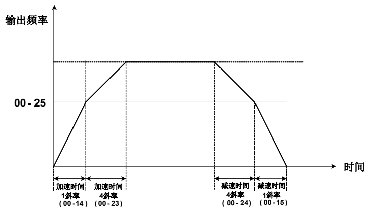
图 4.3.8 自动加/减速切换
