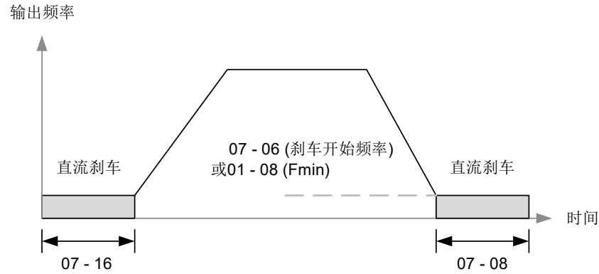
图4.3.54 VF、SLV与SLV2的刹车动作
