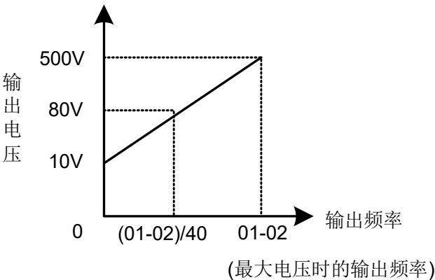
图 4.3.11 输出电压限制曲线
