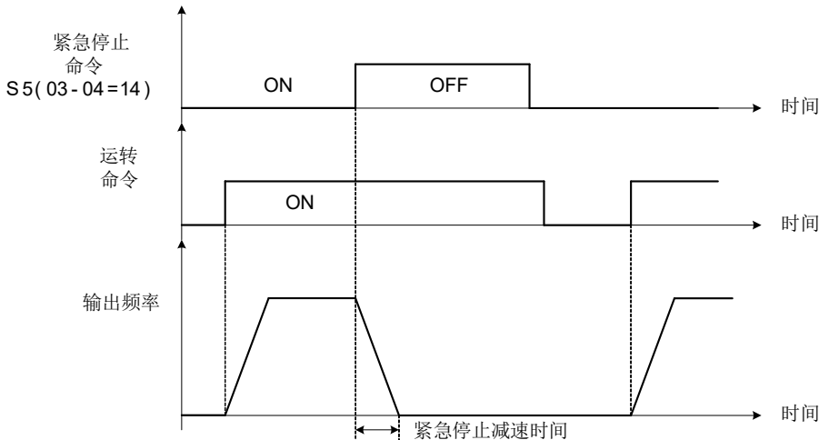
图 4.3.9 紧急停止运转范例
