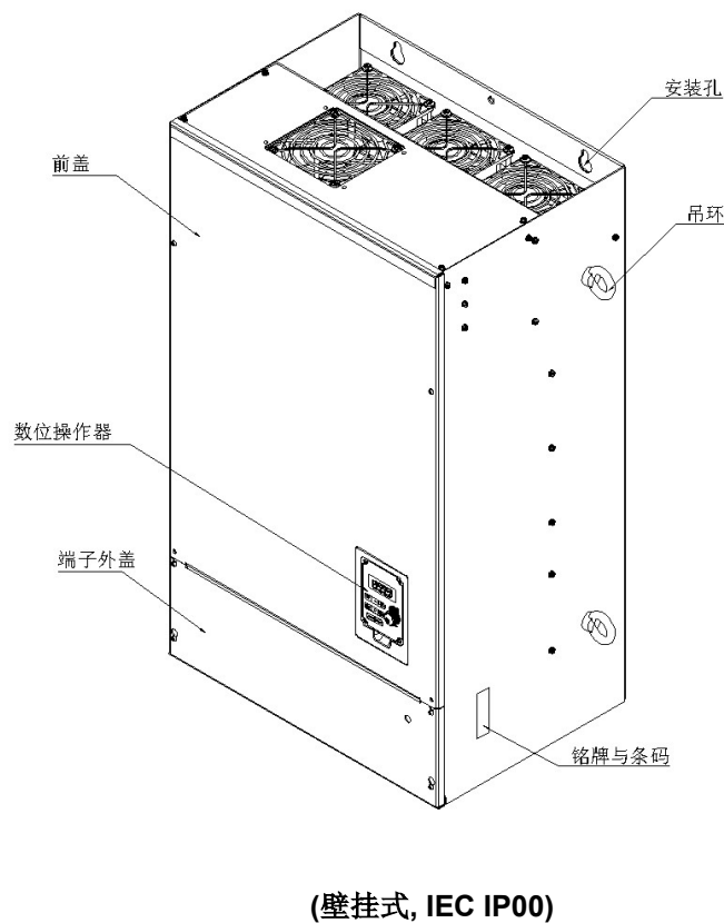
图 3.2 T310 外观图
