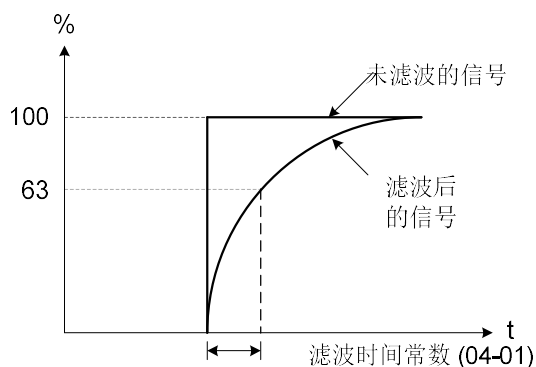
图4.3.34 滤波时间常数
