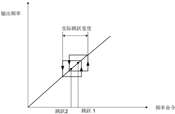
图4.3.84 跳跃频率重叠
