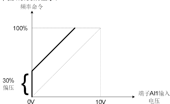
图4.3.38 频率参考偏压调整(范例)
