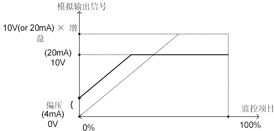
图4.3.48 模拟输出准位调整
