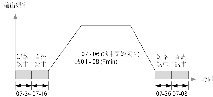
图4.3.57b PMSLV的刹车动作
