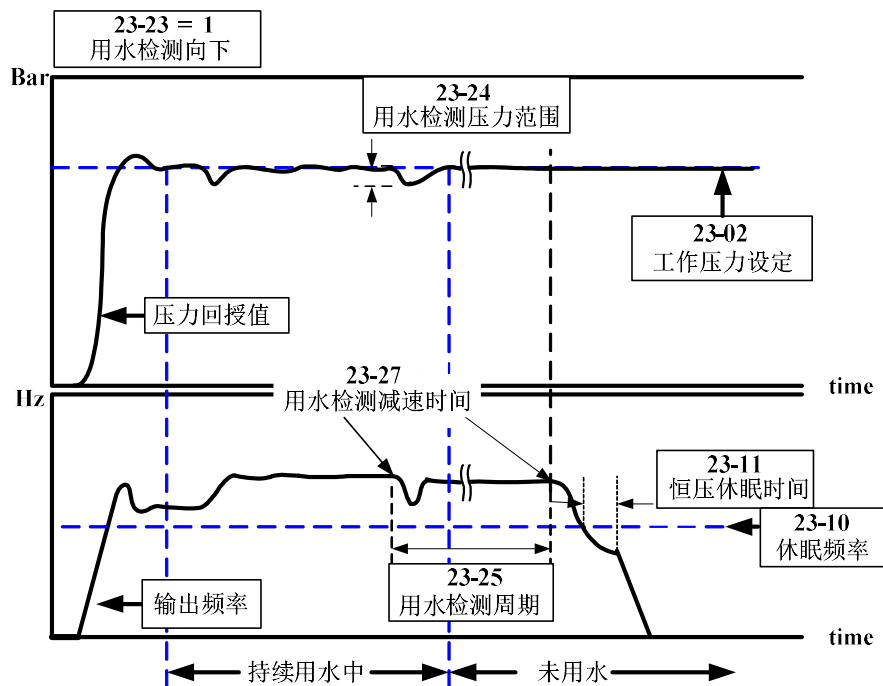
图4.3.108 用水检测向下机能示意图
