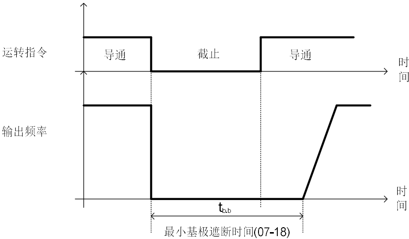
图 4.3.56 自由运转停止
