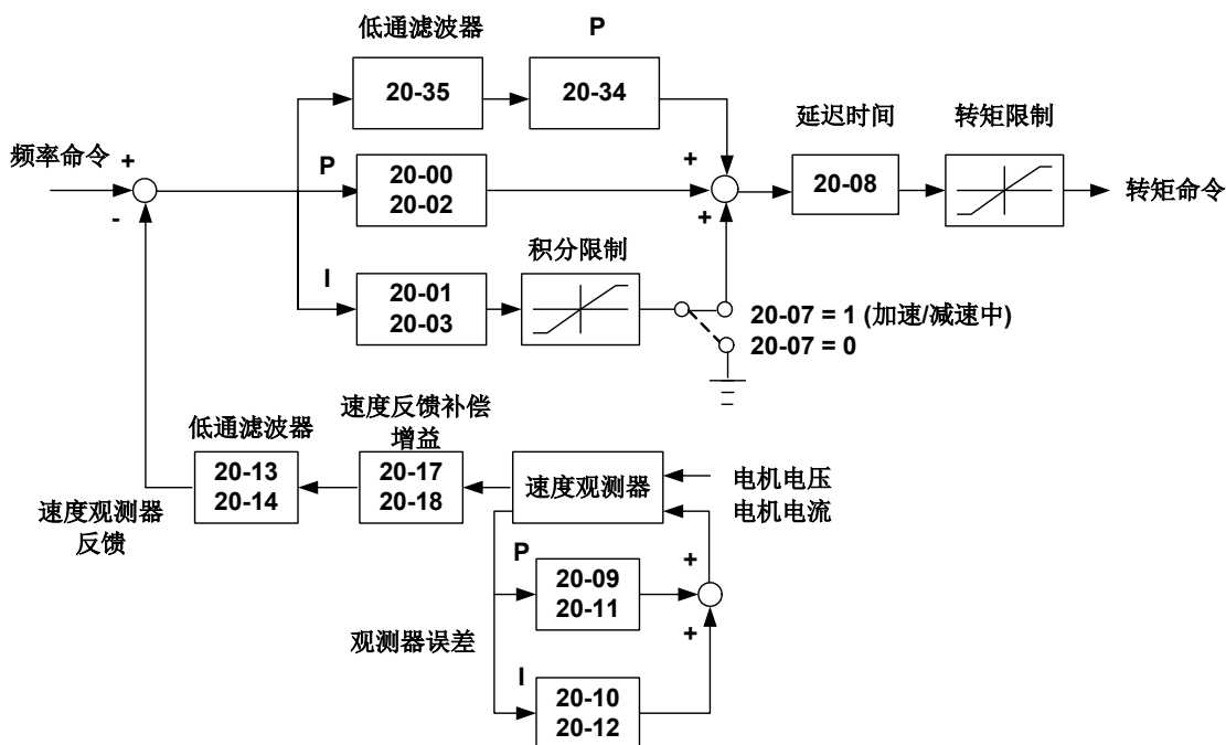
图 4.3.103 速度控制架构(SLV 模式)
