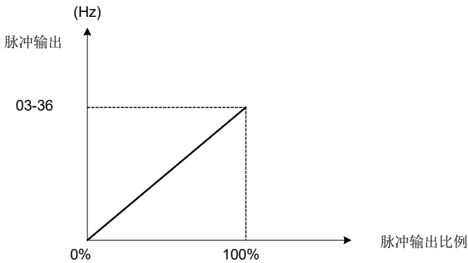
图 4.3.27 脉波输出比例
