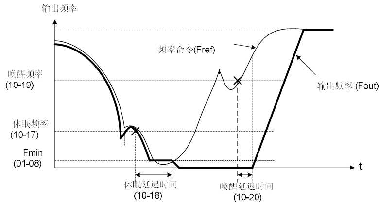
(b) PID 休眠 / 唤醒之时序图
