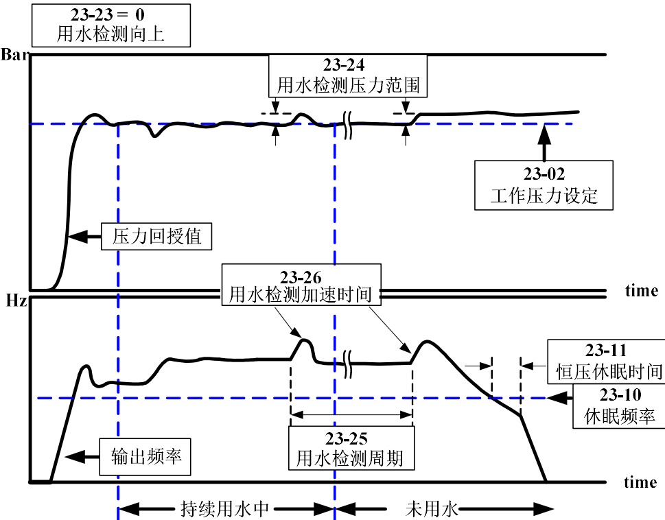
图4.3.107 用水检测向上机能示意图
