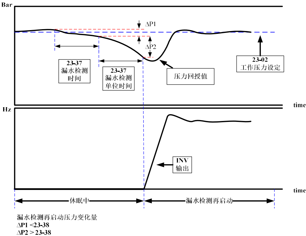
漏水检测 Case1: 压力变化量大于23-38
