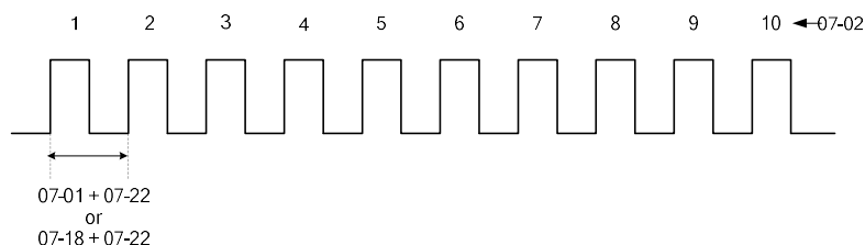
图 4.3.53 自动重启间隔时间
